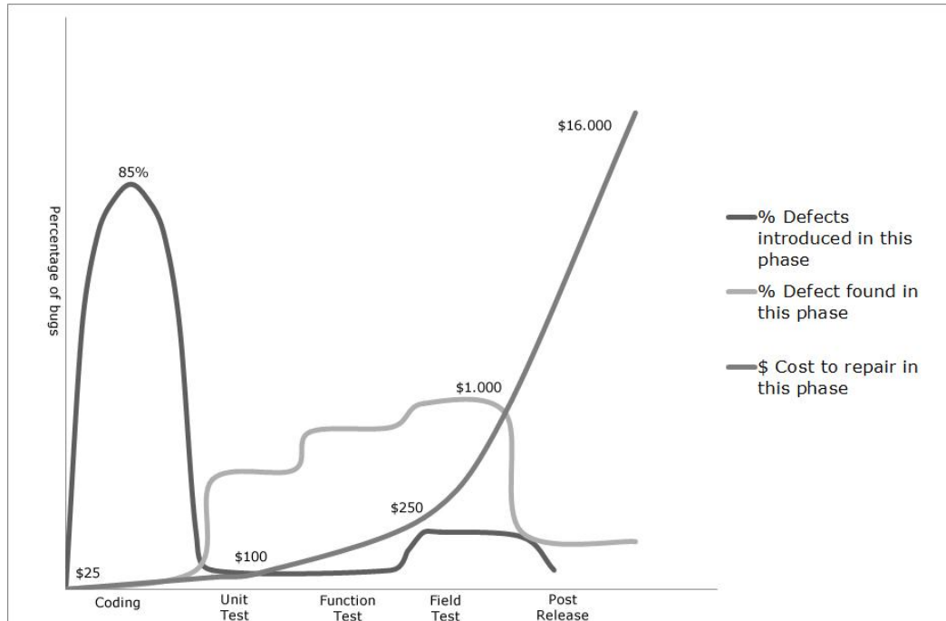
Abbildung 1: Kosten zur Behebung von Sicherheitslücken im Verlauf der Softwareentwicklung [nach: Jo96]
